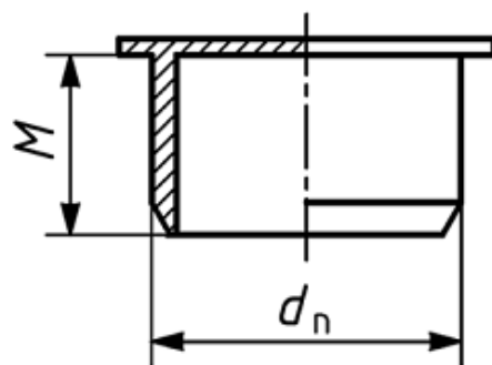
شکل ۱۹- درپوش
