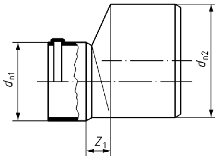
شکل ۱۳- کاهنده
