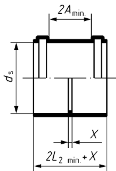
شکل ۱۲- جفت ساز
