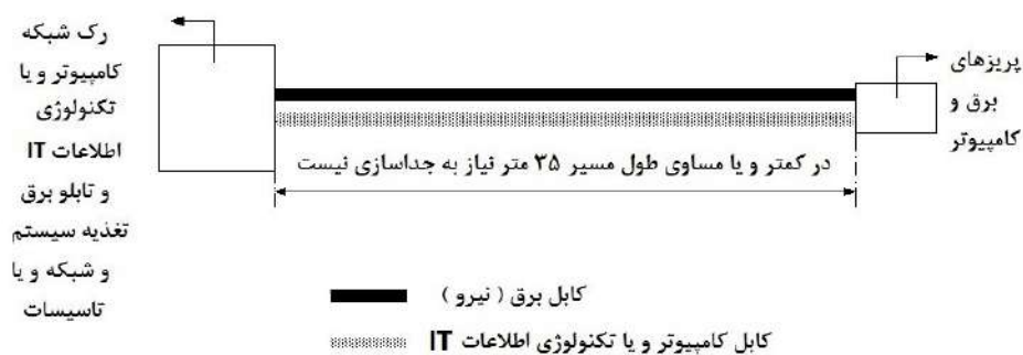
شکل ۱۳-۳-۱۸-۱: طرحواره مسیر مشترک کابل برق و کابل کامپیوتر یا فناوری اطلاعات IT برای طول مسیر کمتر یا مساوی ۳۵ متر
