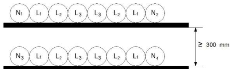
شکل ۷-۱۳-۱-۷-۱:۸ آرایش چسبیده به هم در دو تراز به فاصله ۳۰ سانتی متر از هم برای ۱۲ رشته کابل تک رشته موازی (سه فاز)
