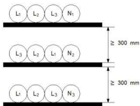
شکل ۷-۱۳-۱-۷-۱:۵ آرایش چسبیده به هم در سه تراز و هر تراز به فاصله ۳۰ سانتی متر از هم برای رشته کابل تک رشته موازی (سه فاز)
