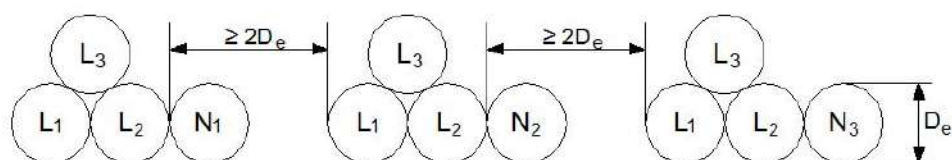
شکل ۷-۱۳-۱-۷-۱:۶ آرایش مثلثی مخصوص برای رشته کابل تک رشته موازی (سه فاز)
