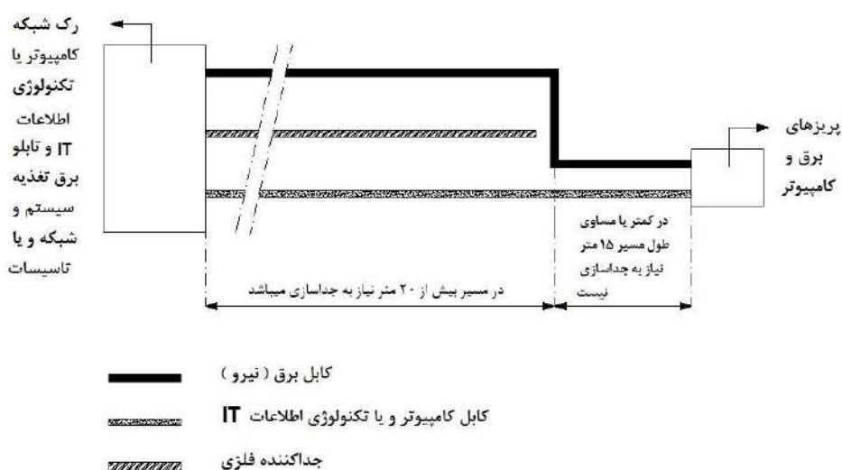
شکل ۱۳-۳-۱۸-۲: طرحواره مسیر مجزا و مشترک کابل برق و کابل کامپیوتر یا فناوری اطلاعات IT برای طول مسیر بیش از ۳۵ متر
