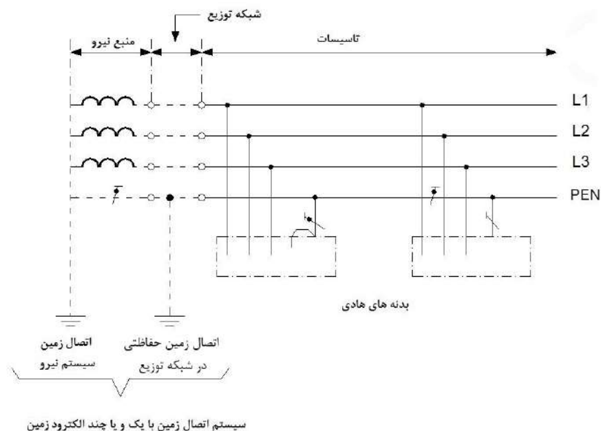
شکل پ ۱-۲:۲ سیستم TN-C در سیستم سه فاز چهار سیمه با هادی مشترک حفاظتی - خنثی در سرتاسر سیستم
