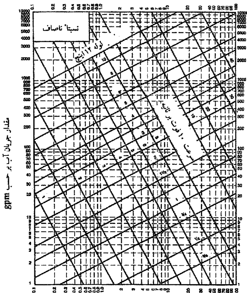
افت فشار آب بر حسب فوت در ۱۰۰ فوت طول
