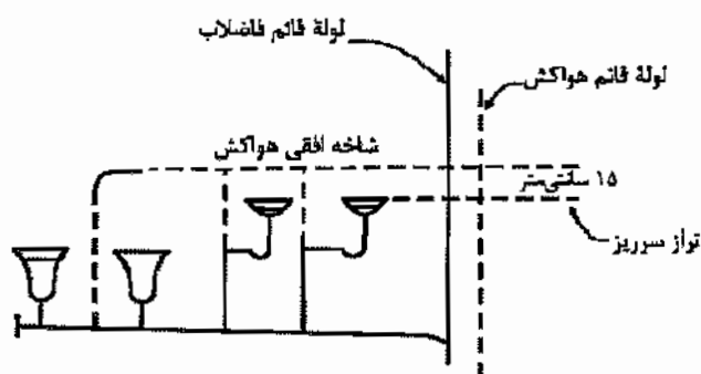
شکل ۱۶-۵-۲-۵ "ب" (۲) - اتصال هواکش به شاخه افقی لوله فاضلاب
