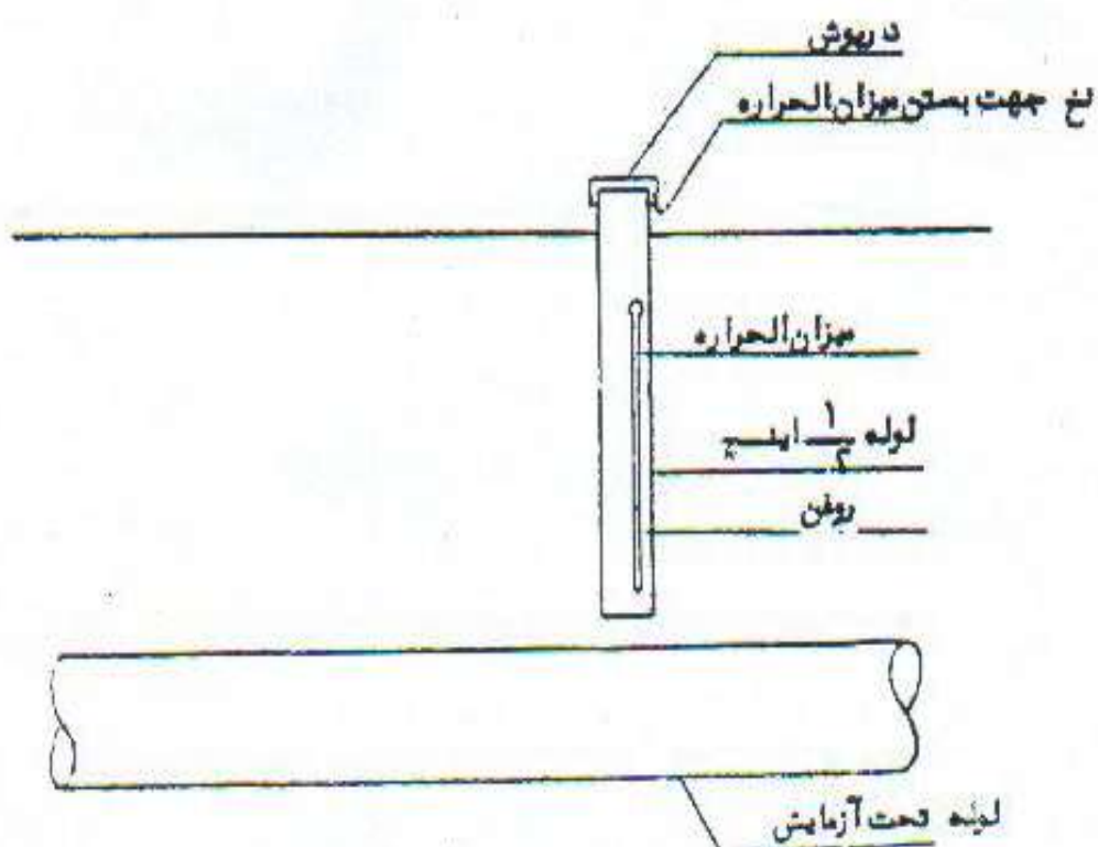
شکل ۲- نحوه نصب میزان الحرارة
